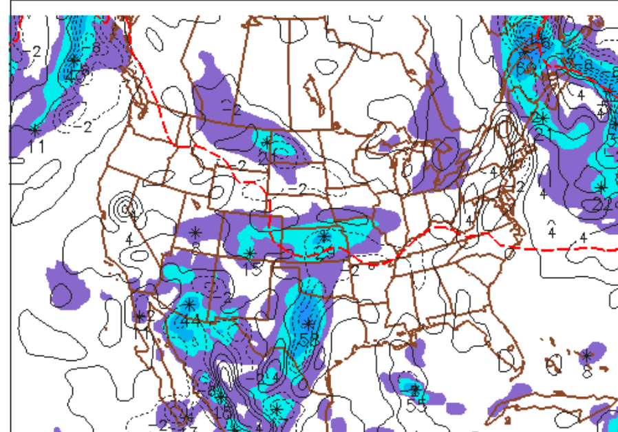
NEMS-NMMb 6HR PRECIP ENDING SUN 150201/0000V054 NEMS-NMMb 700MB OMEGA/850MB QC SUN 150201/0000V054
