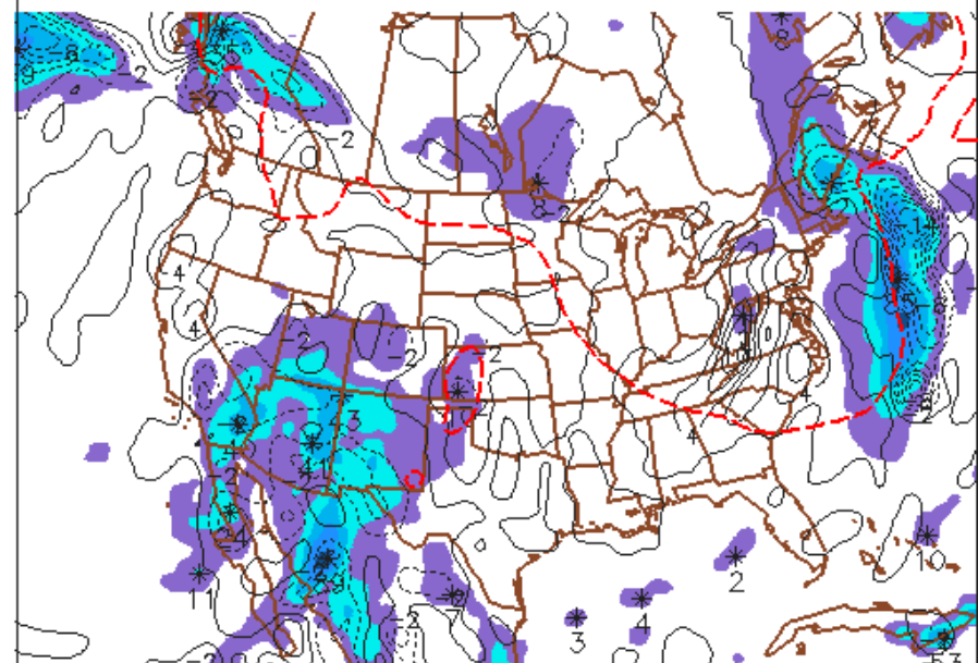
NEMS-NMMb 6HR PRECIP ENDING SAT 150131/0000V030 NEMS-NMMb 700MB OMEGA/850MB OC SAT 150131/0000V030
