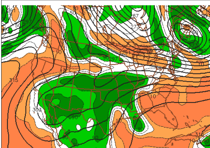
NEMS-NMMb 700MB HGT/RH SUN 150201/0000V054 INITIAL TIME = 150129/1800F054
